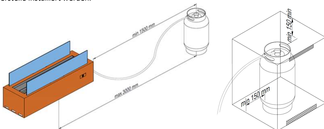
Abbildung 2 – Abstand zwischen der Feuerstelle und Gasflasche sowie Gasflaschenverkleidung
