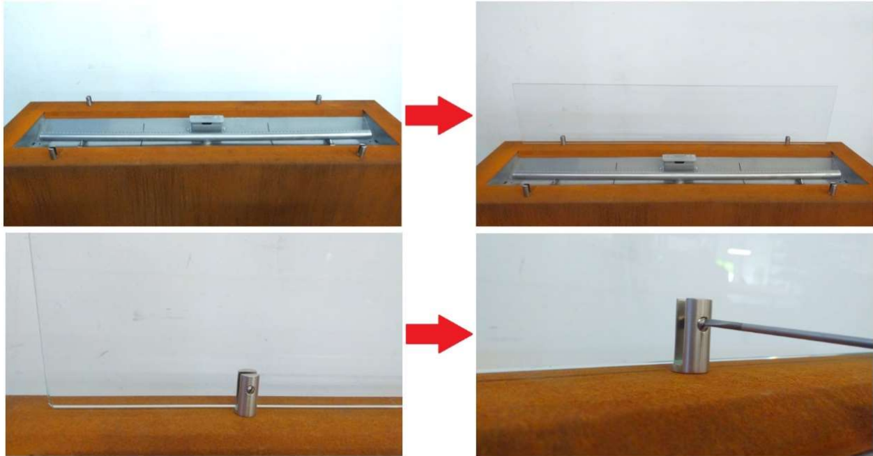
Foto 3 – Montage der Glaspaneel
