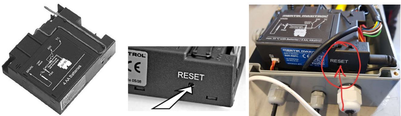
Foto 5: „RESET“-Knopf im Empfängergehäuse
